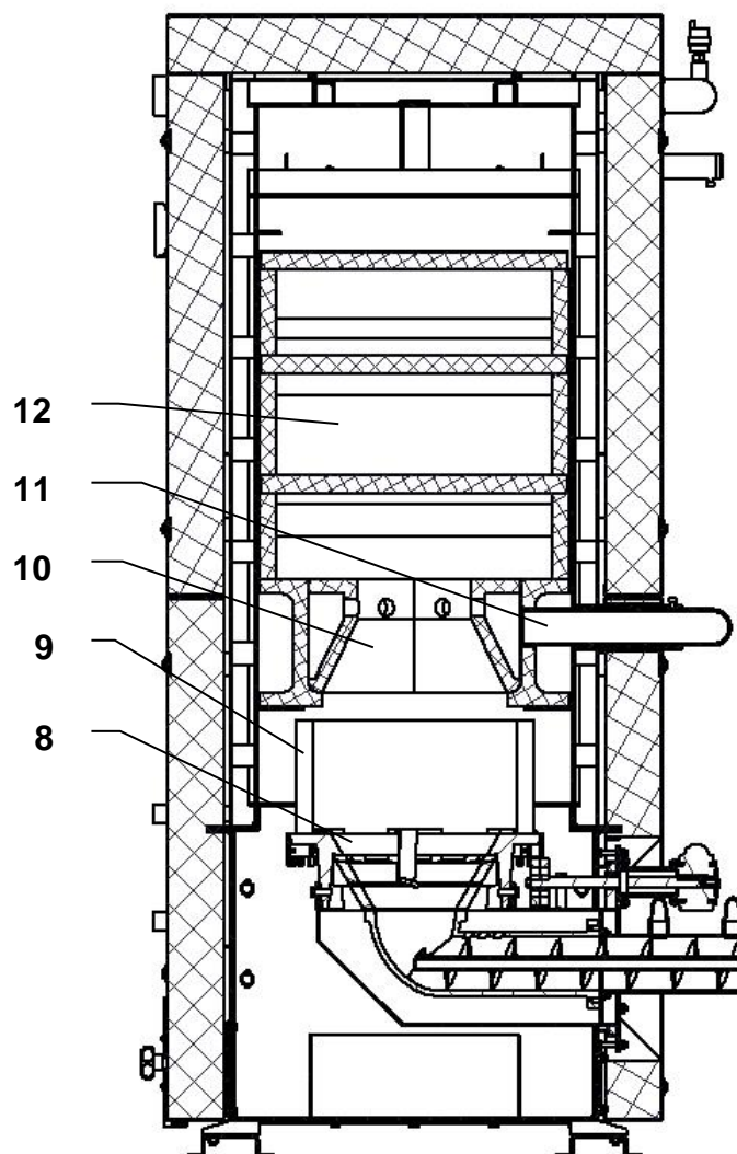
Obr. č. 11 Řez spalovací komorou kotle
