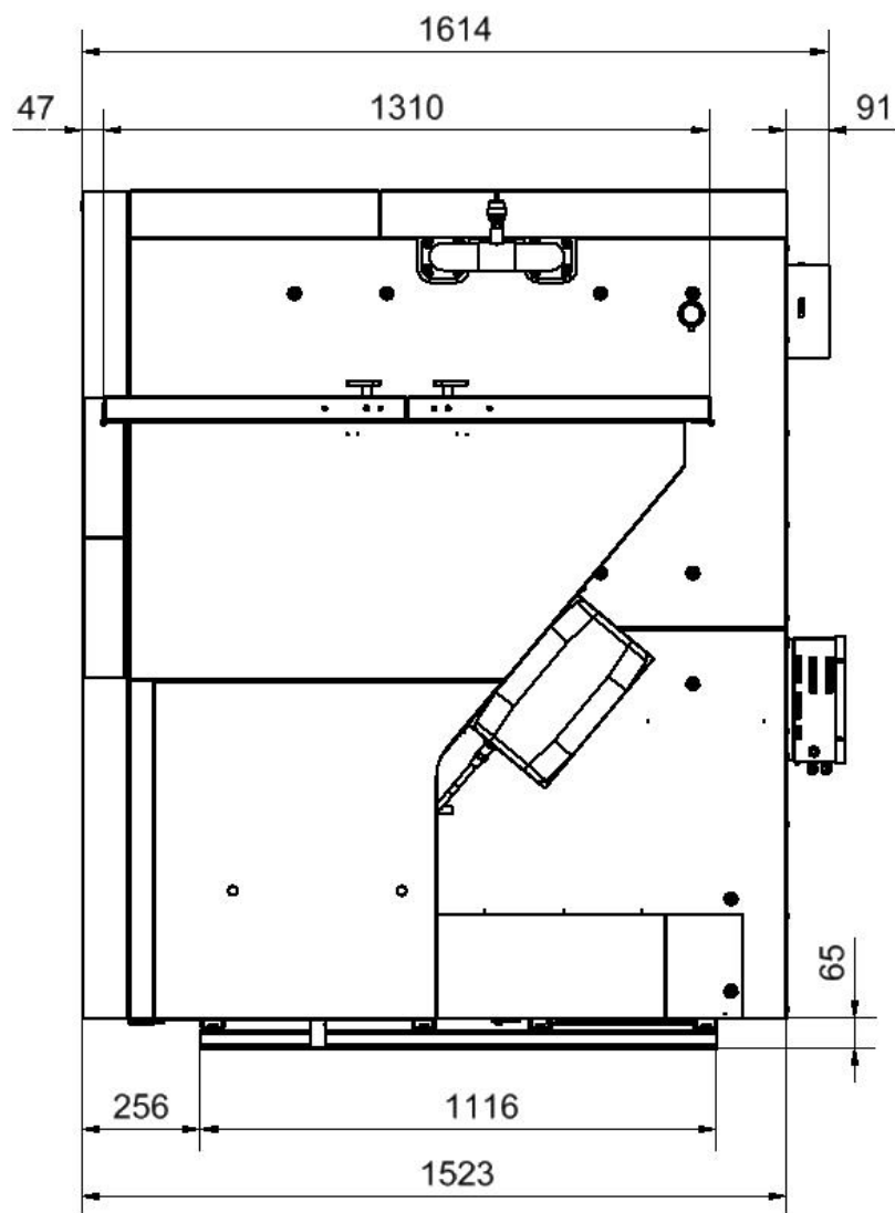
Obr. č. 2 Základní rozměry kotle BENEKOV C77
