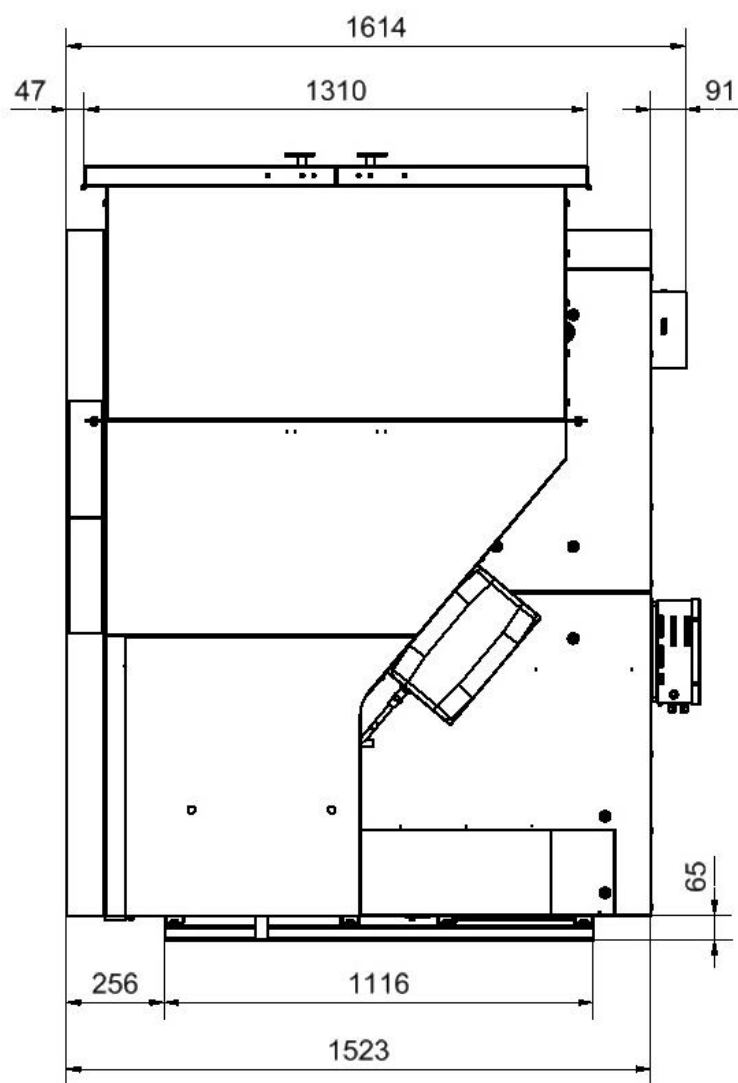
Obr. č. 4 Základní rozměry kotle BENEKOV C77 (s přídatným modulem zásobníku paliva)
